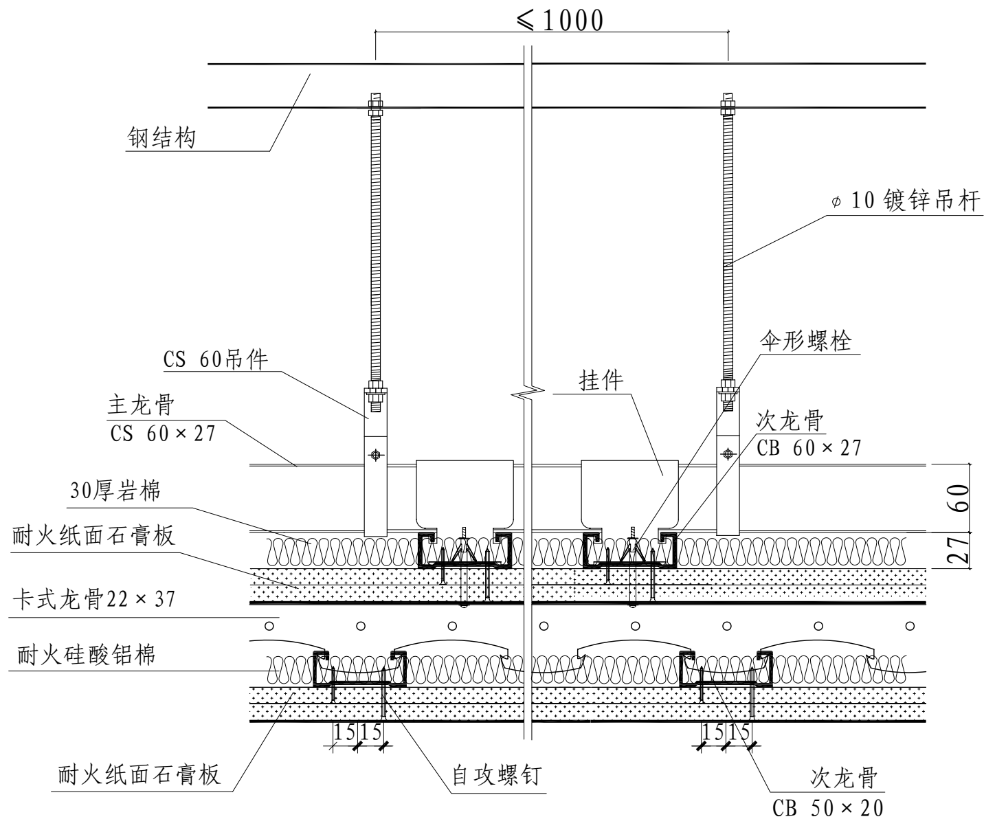
耐火、隔声双层吊顶结构做法详图
